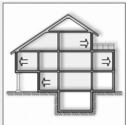
Slika 2 Grafički prikaz elemenata vanjske ovojnice vanjskih zidova grijanog prostora IZVOR: Programski alat KI Expert 2013 v.4.7.0.2.
